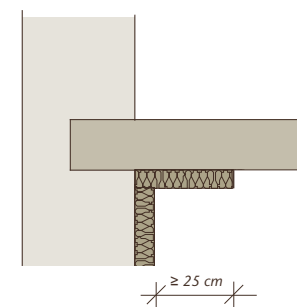
Flankendämmung ggf. bei Beton, bei Lehm oder Ziegel in der Regel nicht
