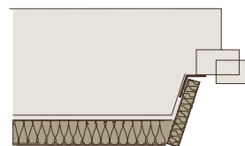
Luftdichtung und Dämmung in der Fensterleibung
