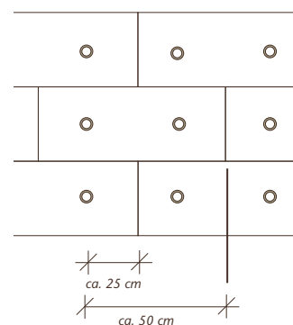
Schraubenabstand, Plattenabstand
