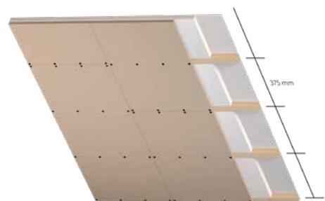
Dakhelling aanzicht
