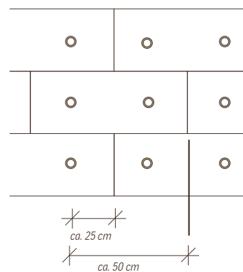
Schroefafstand, plaatafstand
