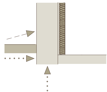
Risico's door andere vochtbronnen
