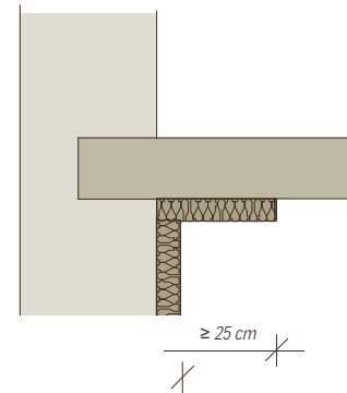
Flankisolatie evt. bij beton, bij leem of baksteen meestal niet
