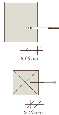
Verankeringsdiepten
