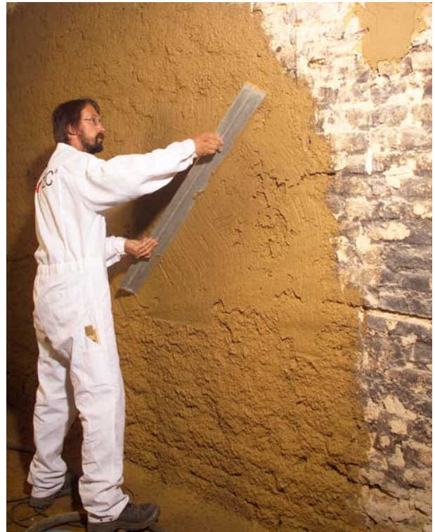
Abbildung 6.1.2: Grobes Abziehen der frischen Putzfläche mit dem Aluminium-Richtscheit
