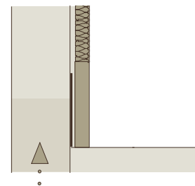
Fußpunkt mit Abdichtung und Schaumglasdämmung
