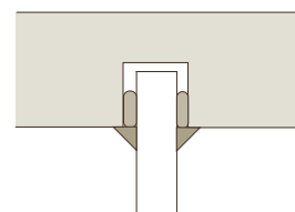
Dichten mit Stopfwolle und Lehmputzmörtel (auf dem Holz ggf. mit Putzträger)
