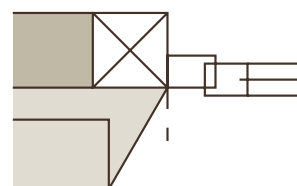
Fensteranschluss \leq 30^\circ
