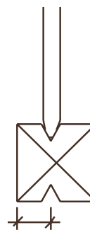
5-6 cm zwischen Außenkante Balken und Mitte Nut
